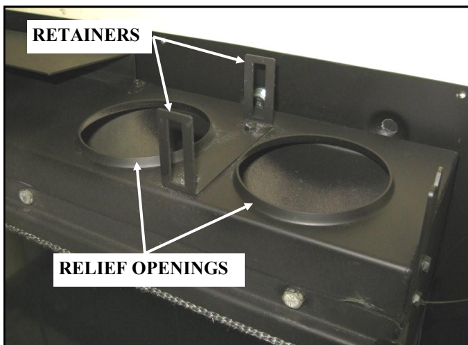
RELIEF DOOR FRONT TAB
